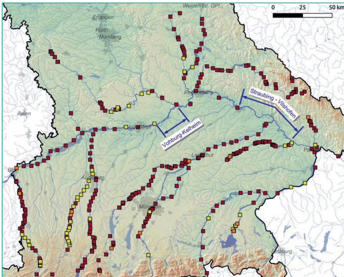
Abbildung 4: Querbauwerke (Stauwerke, Kraftwerke und sonstige Wehre) an der Donau und ausgewählten größeren Seitengewässern; für Donau, Iller, Lech, Wertach, Isar und Inn sind die in der Durchgängigkeit verbesserten Querbauwerke farblich hervorgehoben. Daten: Gewässernetz: DLM1000 © GeoBasis – DE / BKG 2015; Durchgängigkeit: Seifert 2008 und 2009; Höhenrelief: SRTM, Daten des USGS / LP DAAC.
